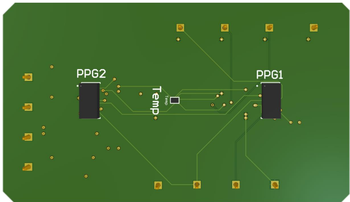
PCB Bottom Layer
