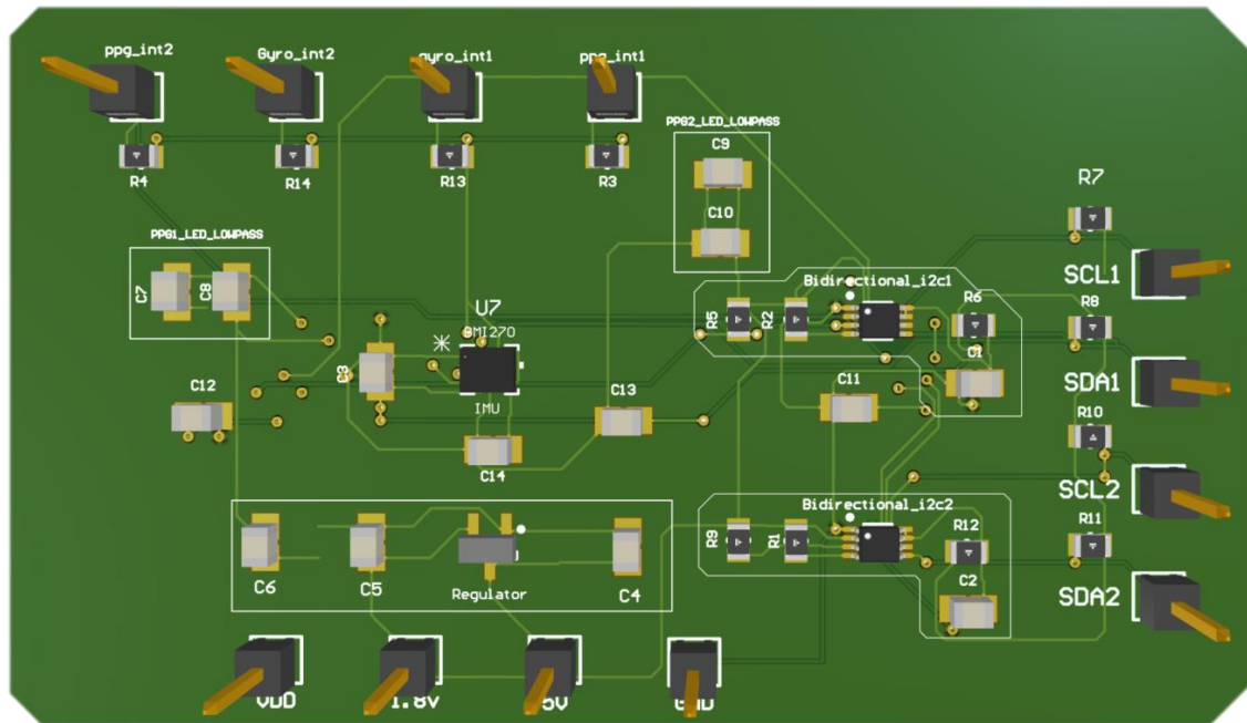
PCB Top Layer
